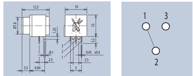
Schaltbild · Wiring Diagram
